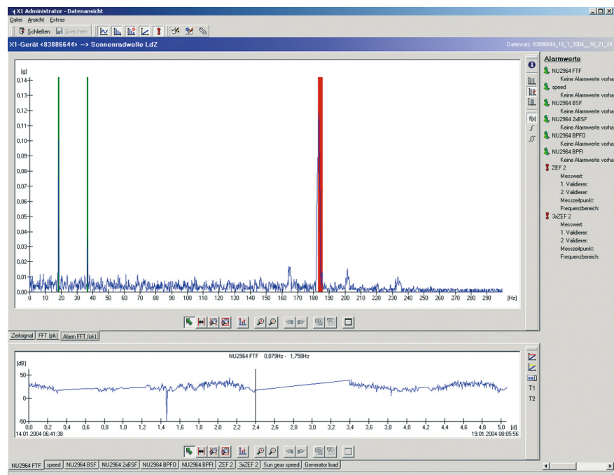
Frequenzselektive Schwingungsüberwachung mit individuell einstellbaren Frequenzbändern
