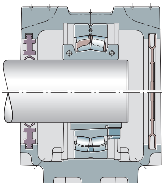
Facile : remplacement de paliers de roulements à rotule sur rouleaux. Même espace de montage pour des roulements à rotule sur rouleaux en deux parties ou des roulements monoblocs avec manchon de serrage
