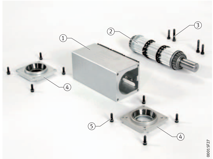
Figura 11 Componentes de la unidad de accionamiento
