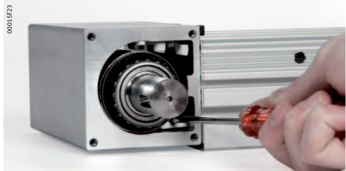
Figura 28 Insertar la correa dentada en la polea dentada
