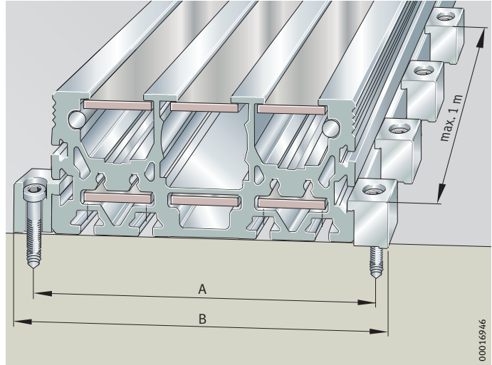
Figura 2 Fijación mediante mordazas de sujeción
