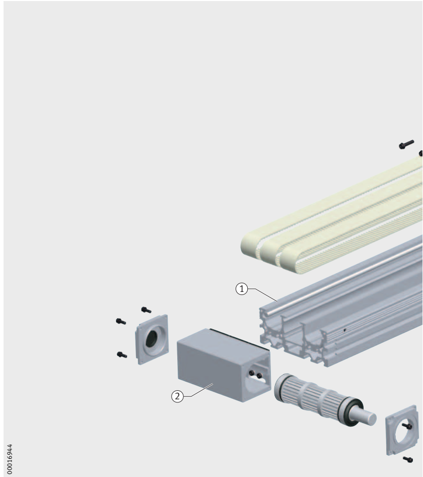
Figura 1 Grupos Módulo lineal MLF1140-3ZR
