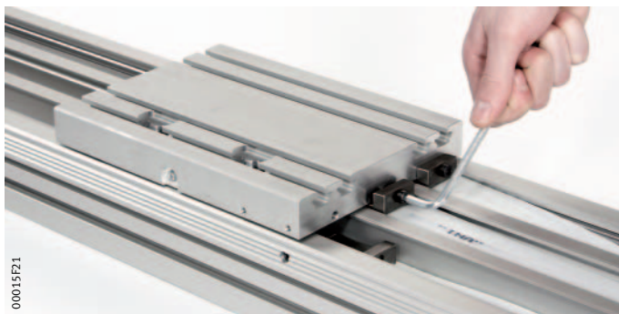
Figura 30 Atornillar el dispositivo tensor al carro
