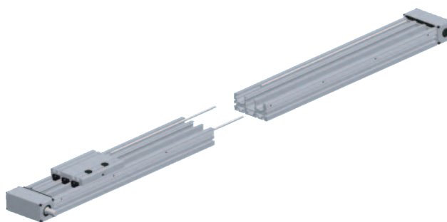
Figura 35 Disponer los tramos de perfil
