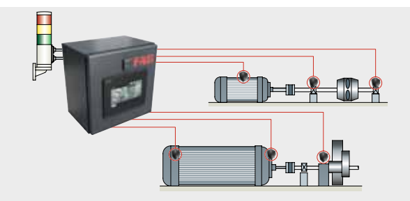
Возможные конструкции с FAG SmartQB
