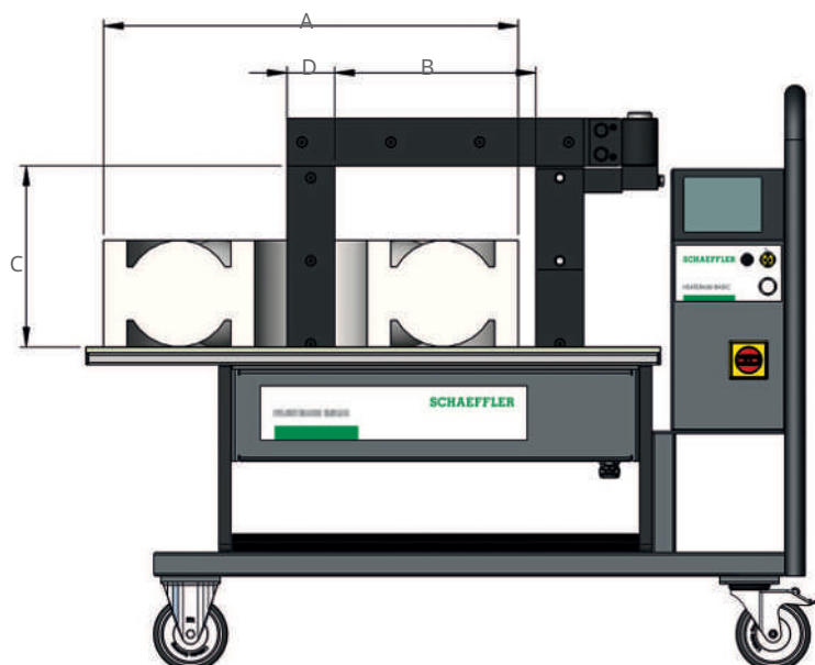
64 Rozmery HEATER400 a HEATER600
