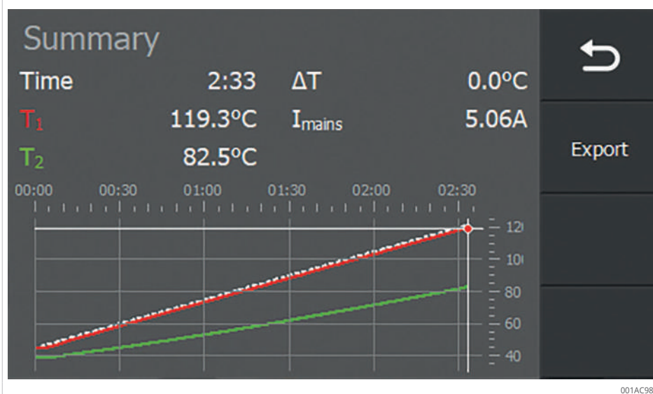
📄 20 Príklad protokolu o ohreve
