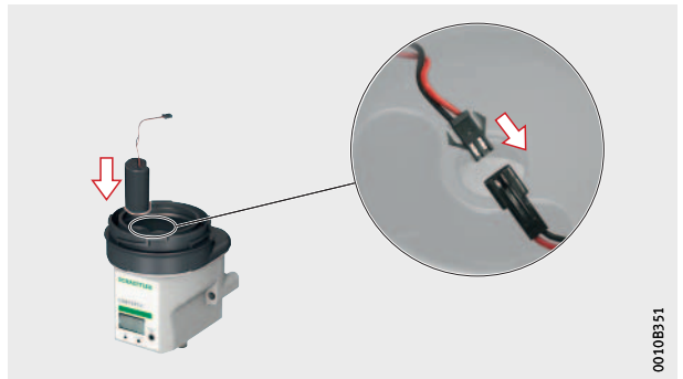
Figura 9 Colocar y conectar la batería
