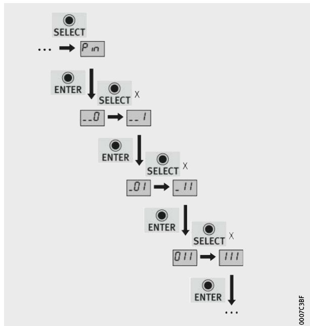
Bild 25 Beispiel Neue PIN: 111
