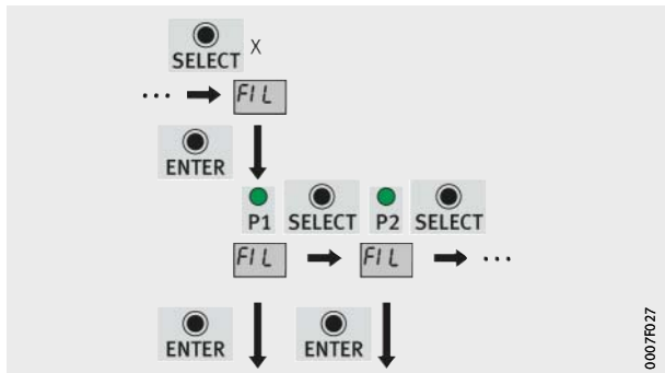
Bild 12 Entlüften der Pumpe
