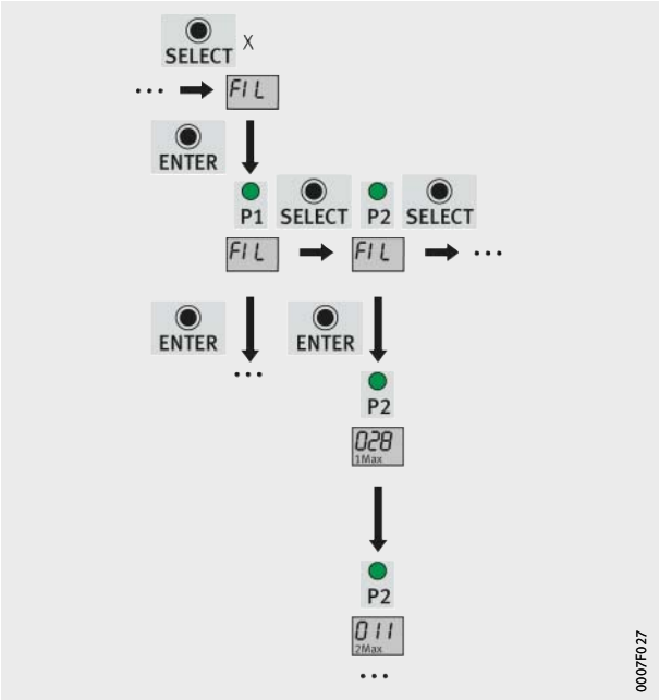
Bild 24 Funktion FIL
