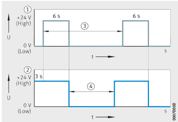
Bild 48 Ansteuerung Pumpenkörper 3
