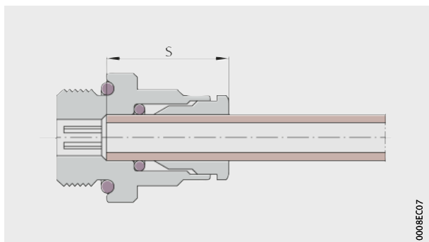
Bild 13 Einstecktiefe
