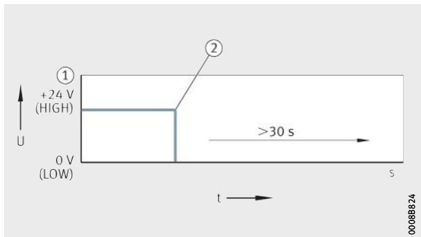
Bild 50 Fehler E1 bis E8
