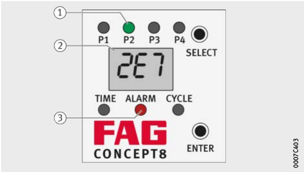
Bild 56 Anzeige Fehler E7
