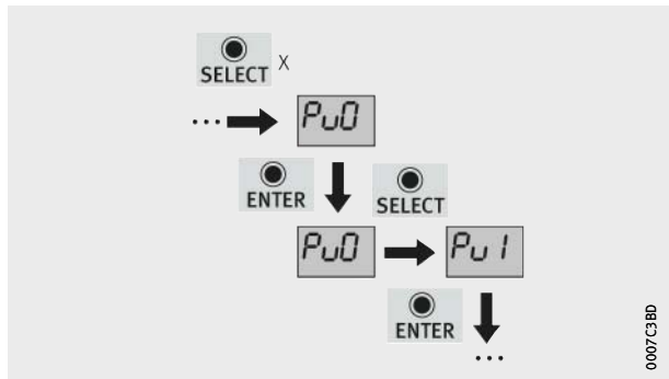
Bild 28 Wechseln der Betriebsart
