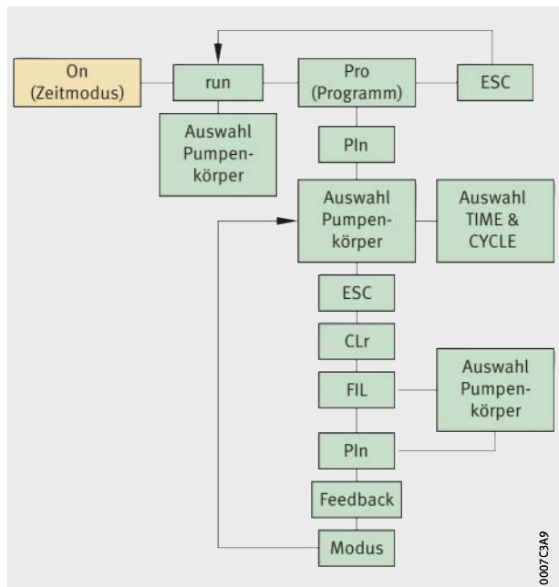
Bild 15 Zeitsteuerung
