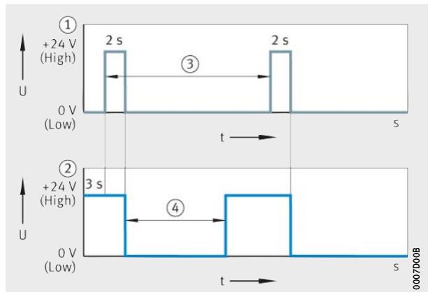
Bild 46 Ansteuerung Pumpenkörper 1
