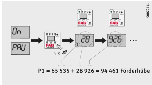
Bild 59 Überlauf
