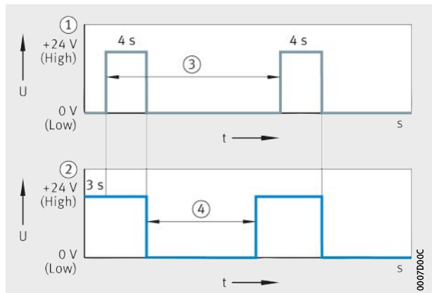
Bild 47 Ansteuerung Pumpenkörper 2
