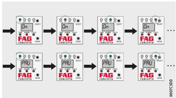
Bild 27 Beispiele Betriebsarten
