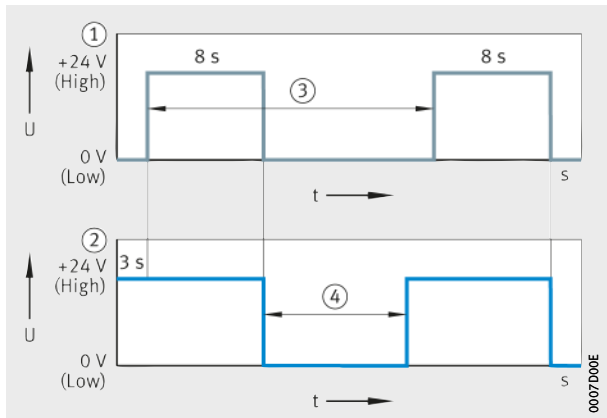
Bild 49 Ansteuerung Pumpenkörper 4
