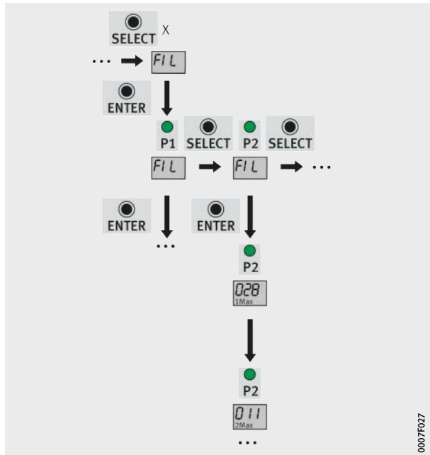
Bild 32 Funktion FIL
