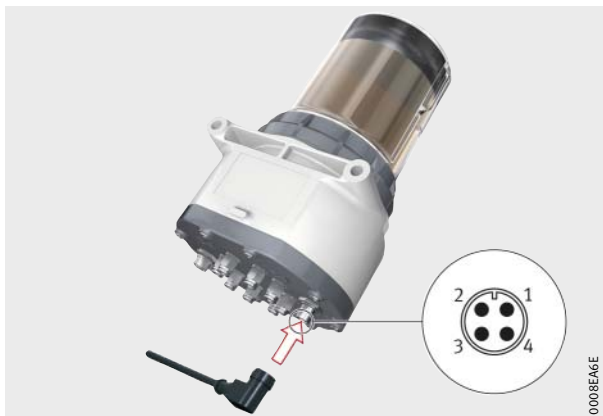
Bild 7 Anschluss FAG CONCEPT8-OIL
