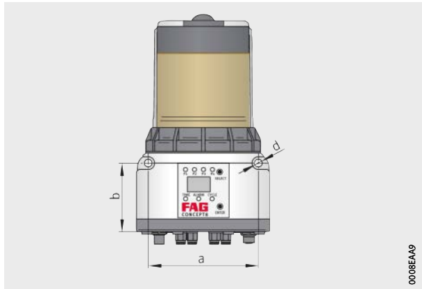
Bild 9 Montagemaße FAG CONCEPT8-OIL
