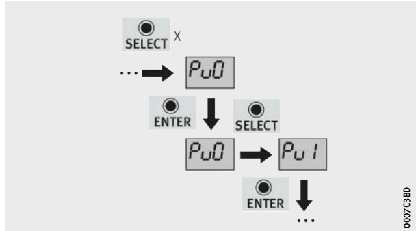
Bild 36 Wechseln der Betriebsart
