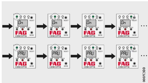
Bild 35 Beispiele Betriebsarten
