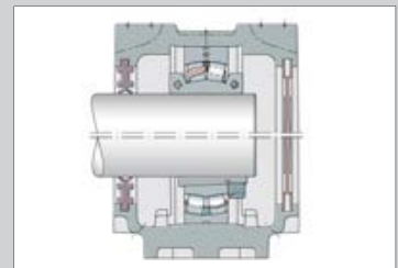
Mismo espacio constructivo para los rdto. partidos oscilantes de rodillos y los no partidos con manguito de fijación
