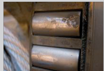
Daños en el elemento rodante de un rodamiento de rodillos cónicos
