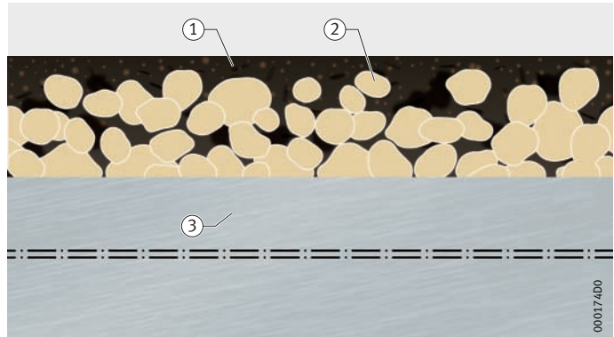
Bild 1 Wartungsfreies Gleitlagermaterial E420-S
