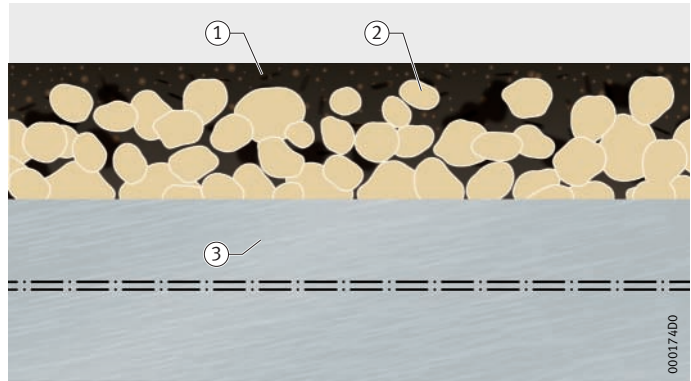
Bild 1 Wartungsfreies Gleitlagermaterial E40-S
