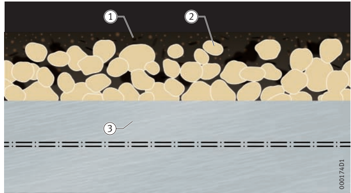
Bild 1 Wartungsfreies Gleitlagermaterial E420
