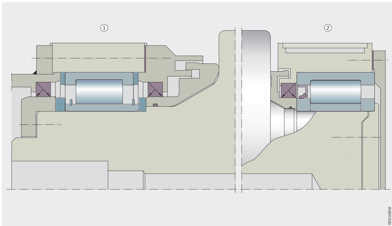
Рисунок 2 · Подшипниковые опоры ролика МНЛЗ ① Свободная опора, ② Фиксированная опора
