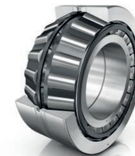
2-Roulement à rouleaux coniques à disposition en X
