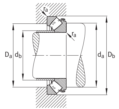
Dimensioni delle parti adiacenti 293...-E1, 294...-E1
