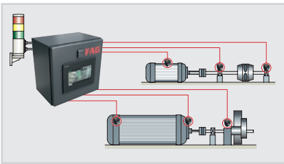
Posible configuración con FAG SmartQB
