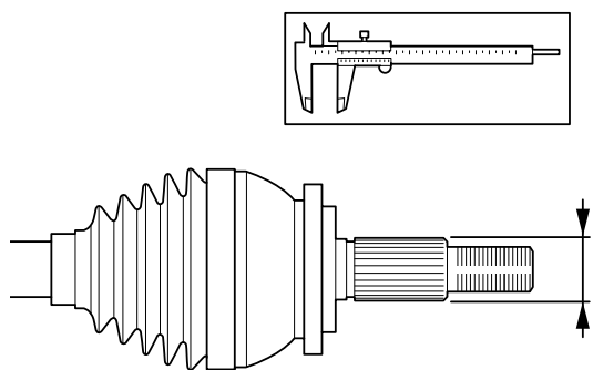
Fig. 1: Om het juiste wiellager te bepalen, moet de buitendiameter van de aandrijfas worden gemeten
